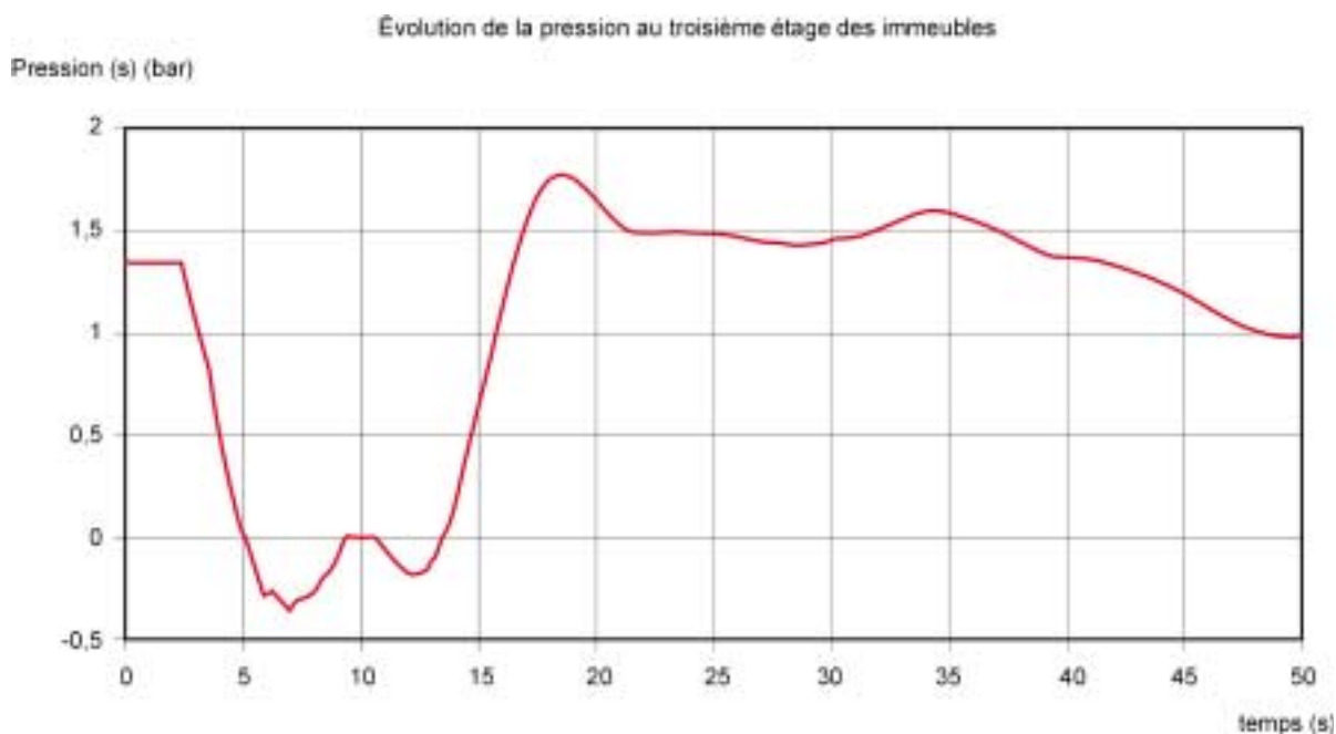
Figure 16 – Disjonction d'une pompe avec un ballon de 2 m 3
