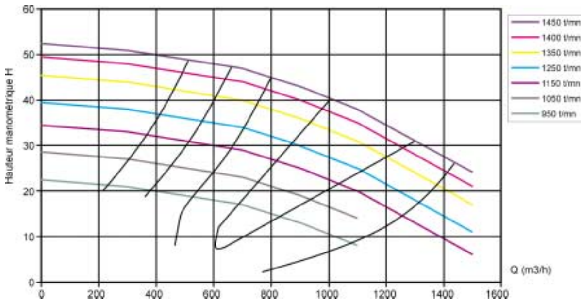
Figure 3 – Courbes caractéristiques d’une pompe à vitesse variable
