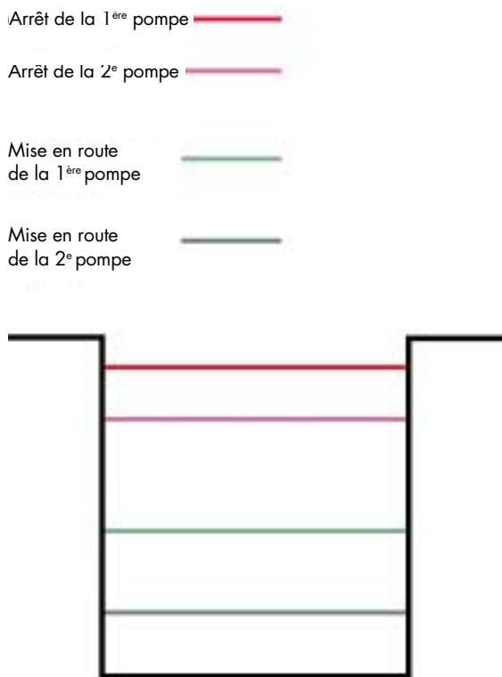
Figure 2 – Exemple d'indexation de pompes sur les niveaux dans un réservoir
