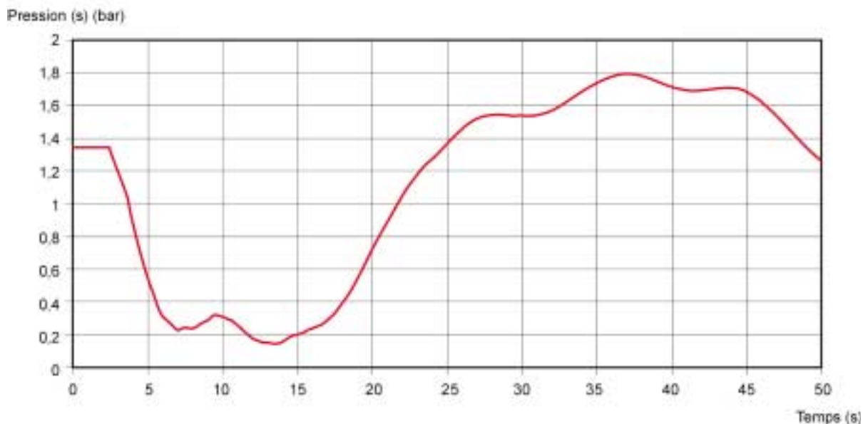
Figure 17 – Disjonction d'une pompe avec deux ballons de 2 m 3 chacun
