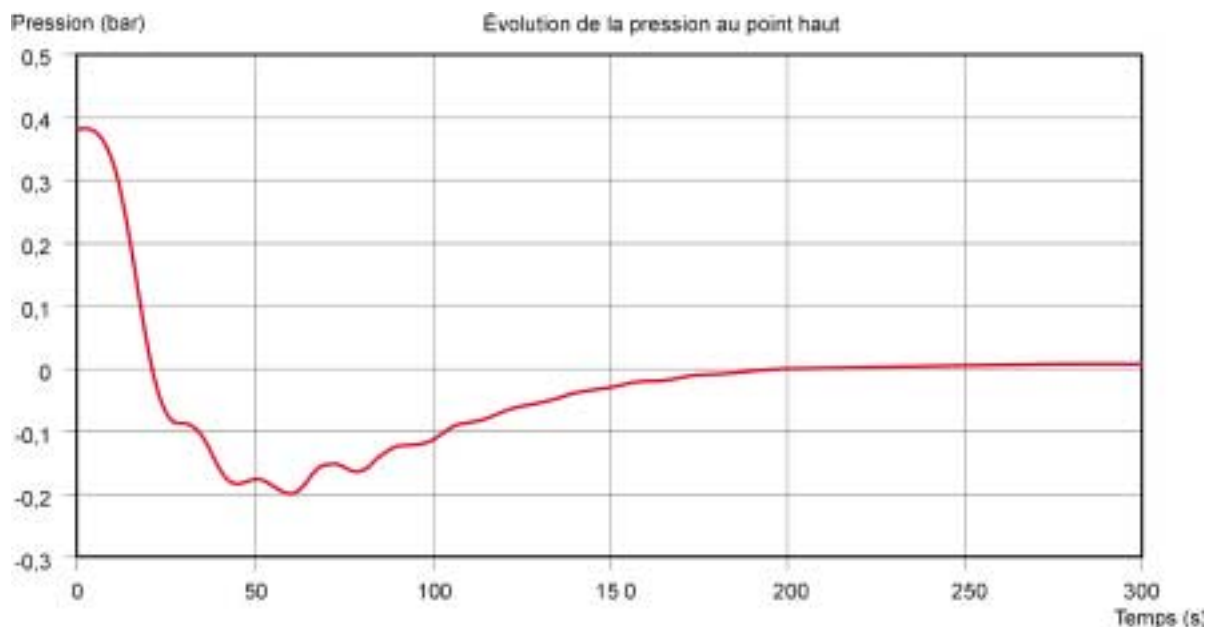
Figure 13 – Ouverture simultanée des trois vannes en situation actuelle
