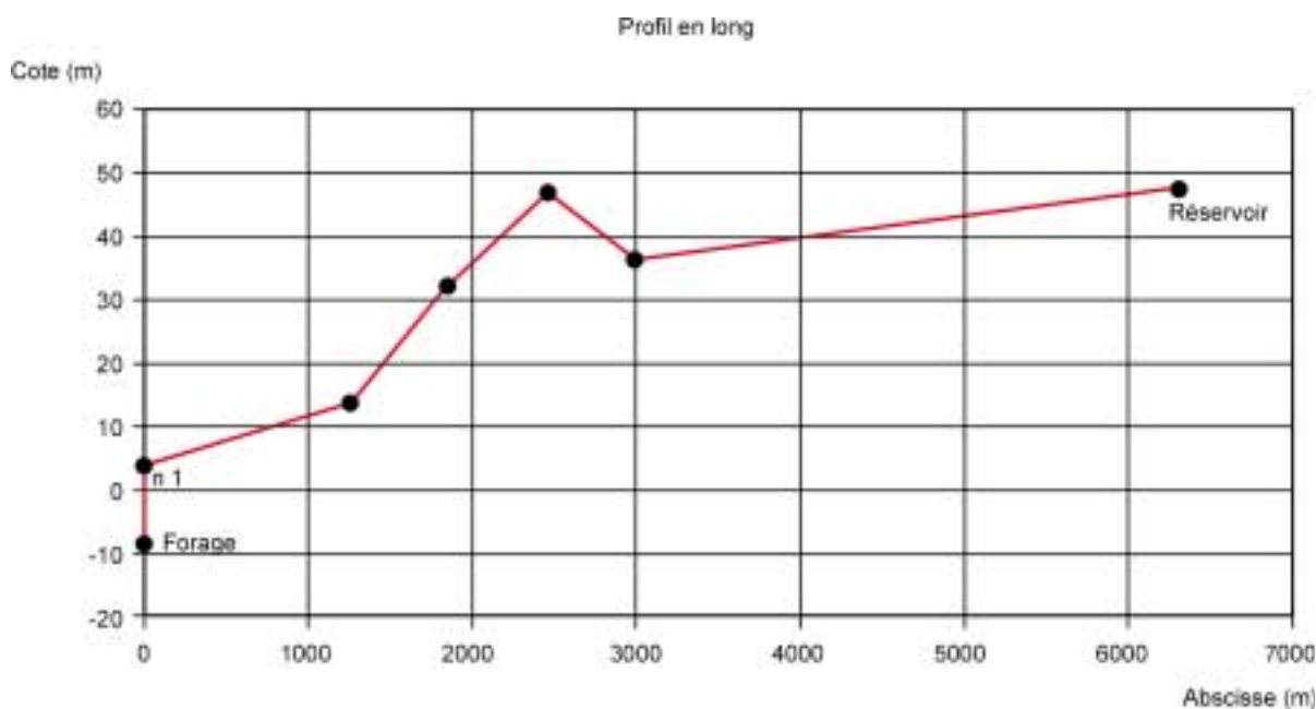
Figure 15 – Profil en long de la conduite principale
