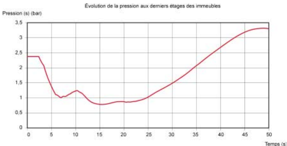
Figure 19 – Disjonction des deux pompes avec un ballon de 4 m 3 en plus du ballon de 2 m 3
