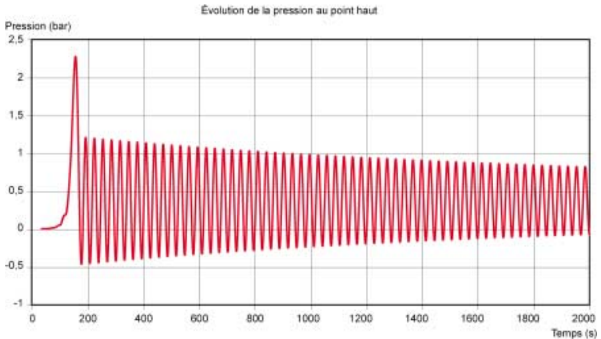
Figure 11 – Fermeture simultanée des trois vannes en situation actuelle
