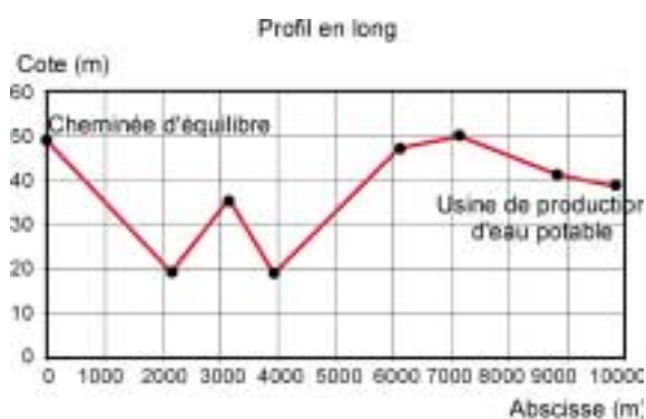
Figure 10 – Profil en long de la conduite à protéger
