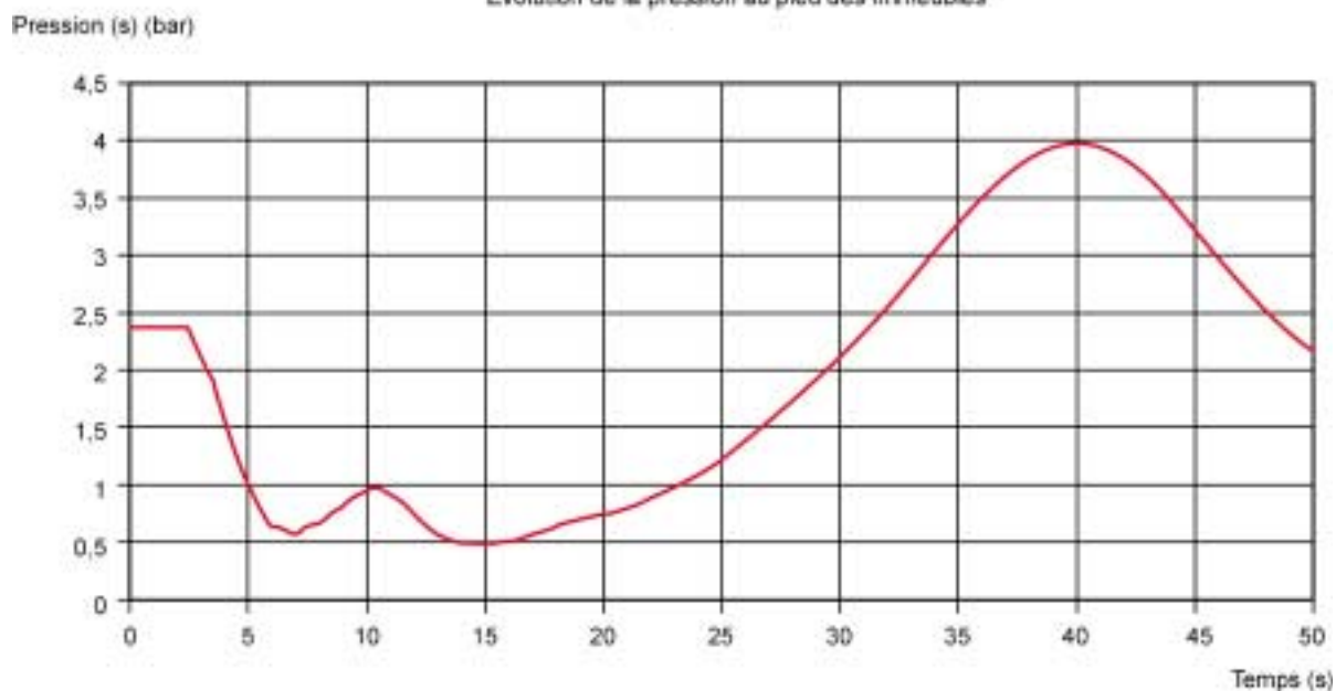
Figure 18 – Disjonction des deux pompes avec une protection de deux ballons de 2 m 3 chacun
