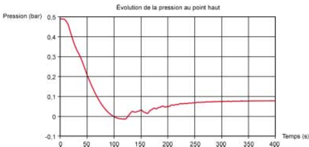
Figure 14 – Ouverture simultanée des trois vannes en six minutes avec un plan d'eau dans la cheminée d'équilibre à 55 m
