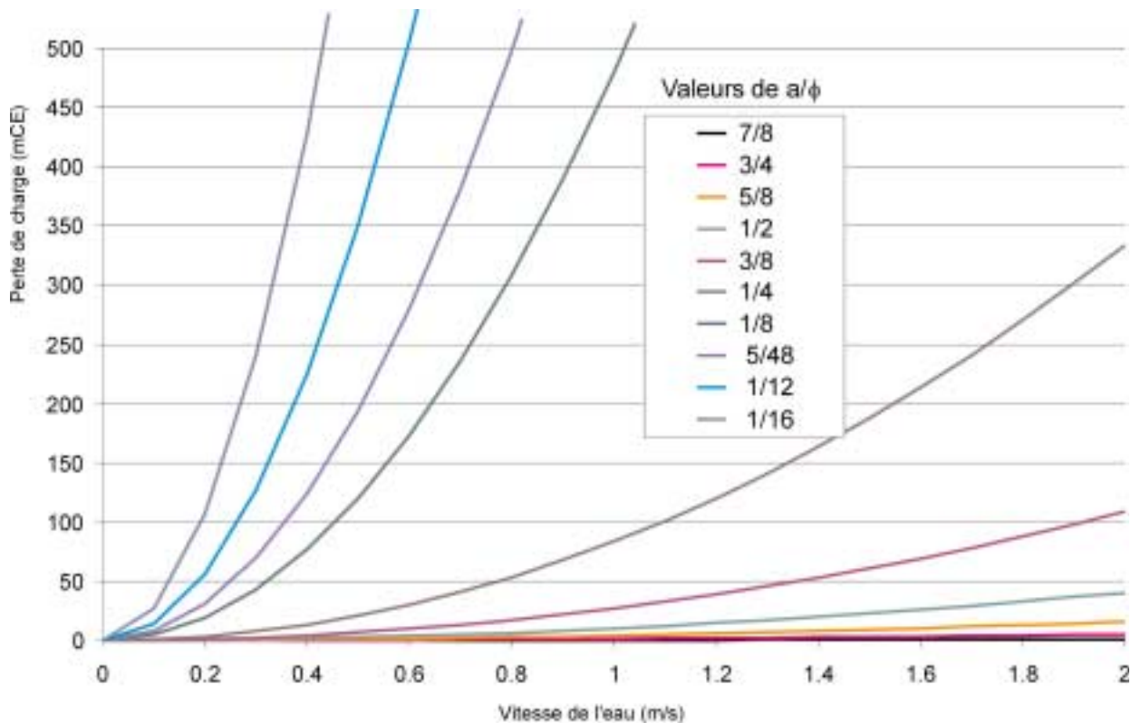
Figure 8 – Courbes de pertes de charge pour chaque degré de fermeture d'une vanne à opercule
