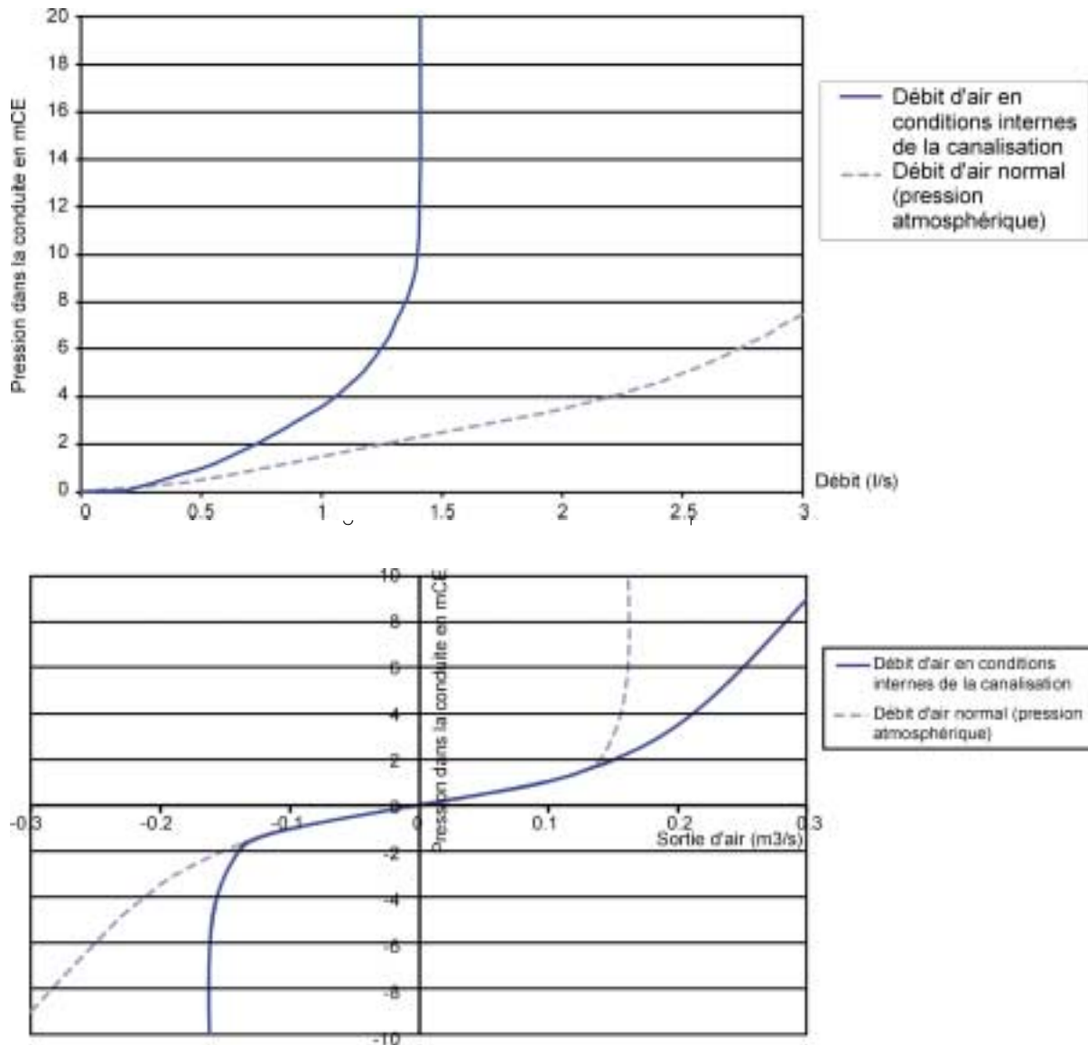
Figure 5 – Entrée et sortie d'air à grand débit
