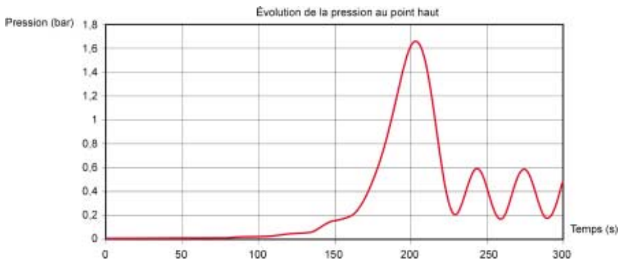
Figure 12 – Fermeture simultanée des 3 vannes en 4 minutes
