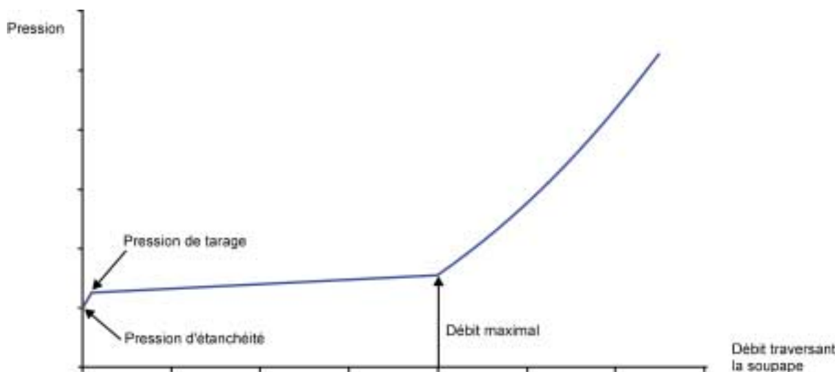
Figure 6 – Caractéristique d'une soupape
