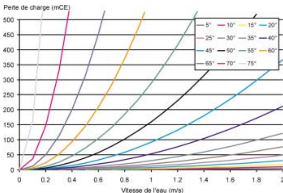
Figure 7 – Courbes de pertes de charge pour chaque degré de fermeture d'un robinet à papillon
